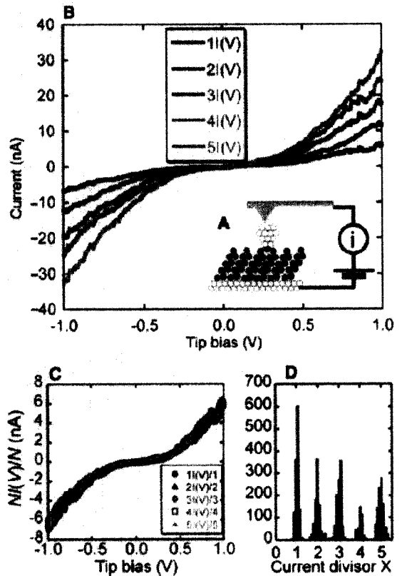
그림 8. 나노 입자/octanedithiol/Au 구조로 C-AFM 방법으로 측정된 전류-전압 결과. (A) 실험 설명도. (B) 대표적 다섯 개의 전류-전압 곡선. (C) (B)의 결과를 정수로 나누었을. (D) 나누는 약수의 histogram. Reprinted from [25], X. D. Cui et al., Science, Vol. 294, p. 571 (2001).
